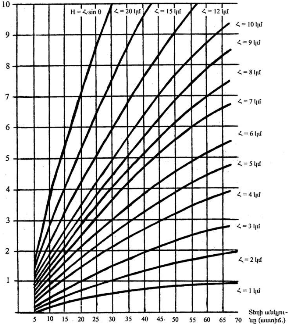
Նկ. 2 Բարձրության որոշման աղյուսակը և գրաֆիկը
