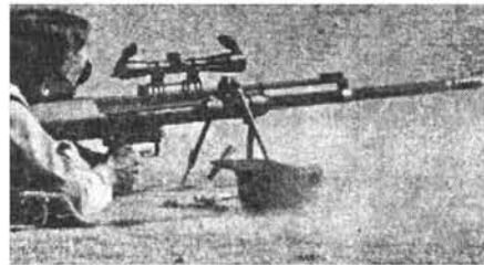
50/12 SU4 մակնիշի 12,7-մմ դիպուկահարական հրացան
