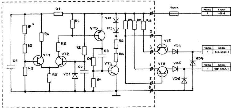
ԼԿ-ՀԱՅ-001 կարգավորչի սկզբունքային սխեման
