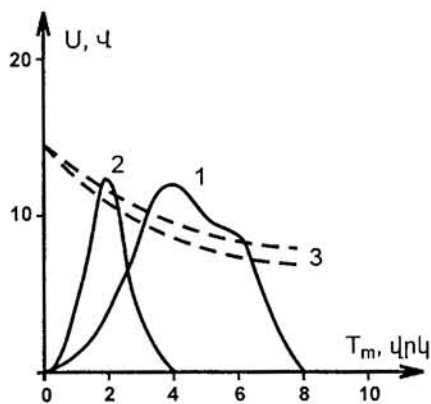
Նկ. 2. Հաստիքային և նորաստեղծ գններատորների փորձարկման արդյունքները
