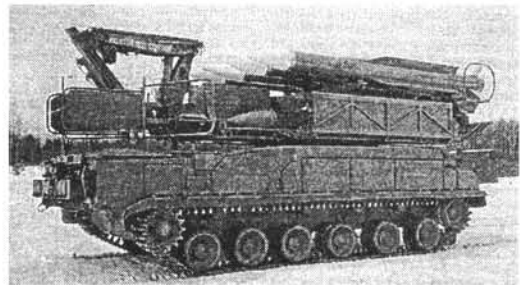
«Բուկ-Մ1» ՋՀՀ արձակման-լիցքավորման 9Ա39 կայանք՝ փնված 9Մ38 ՋԿՀ-ներով
