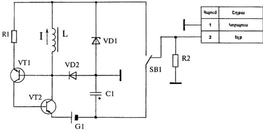
Նկ. 1. ՄՊԳ-9 հաստոցային հավատանկային նունականետի էլեկտրոնային գեներատորի առաջարկվող սկզբունքային սխեման
