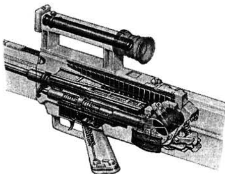
Գ11 ակոսավոր հրացանի կառուցվածքային պատկերը
