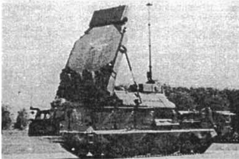
U-300Վ համալիրի հրթիռների ուղղորդման բազմաուղի կայանը
