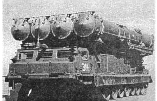
U-300Վ համալիրի 9Ա83 արձակման կայանըը մարտադրավայրին վիճակում
