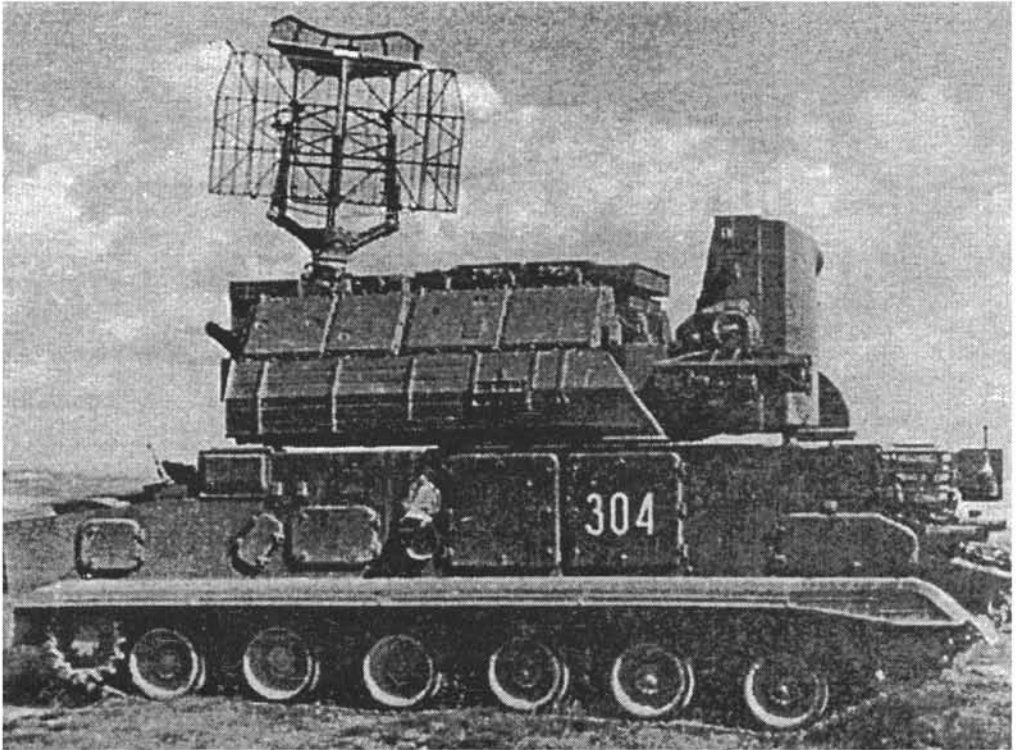
9A330 ՋՀՀ («Տոր-Մ1»)-ի 9Ա330 մարտական մեքենա
