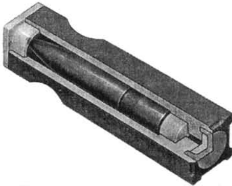
4,7x33 «գինամիտ-նոբել» անպարկուճ հեռադիտակային փամփուշտի կառուցվածքը
