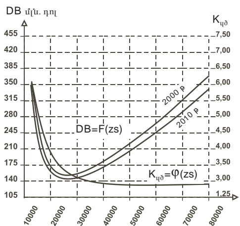
Նկ. 4. Պաշտպանության վրա կատարվող ծախսերի (DB) և K_{40} գործակցի կախումը ՋՈՒ-ի թվաքանակից (ZS) մինչև 2010 թ. տնտեսության վարգայման իրատեսական սցենարի դեպքում
