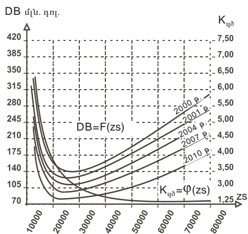
Նկ. 3. Պաշտպանության վրա կատարվող ծախսերի (DB) և K_{40} գործակցի կախումը ՋՈՒ-ի թվաքանակից (ZS) մինչև 2010 թ. տնտեսության վարգայման հոռետեսական սցենարի դեպքում
