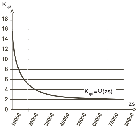
Նկ. 1. K_{\text{փժ}} գործակցի կախումը փինժած ուժերի թվաքանակից ( ZS ) 1-ին դասի համար պարամետրների միջին արժեքների դեպքում
