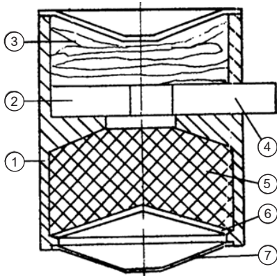
Նկ. 3. Ինքնանշանառվող մարտական տարրի տեղաբաշխումային գծապատկեր
