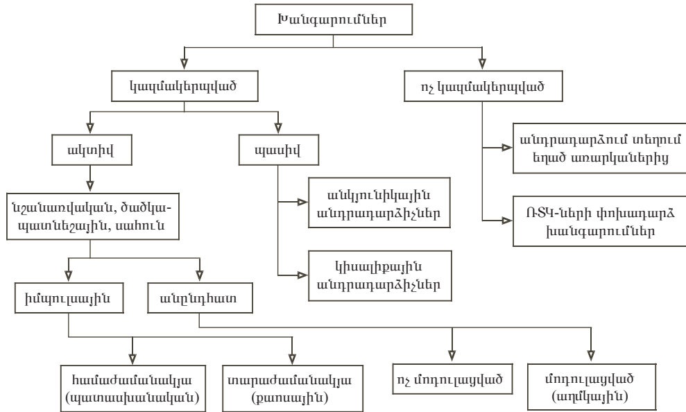
Նկ. 1. Խանգարումների դասակարգման սխեմա
