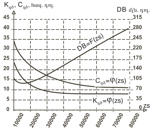
Նկ. 2. K_{\text{փժ}} գործակցի, պաշտպանության համար կատարվող ծախսերի ( DB ) և մեկ փինժառայողի պահման արժողության ( C_{\text{փժ}} ) կախումը փինժած ուժերի թվաքանակից ( ZS )
