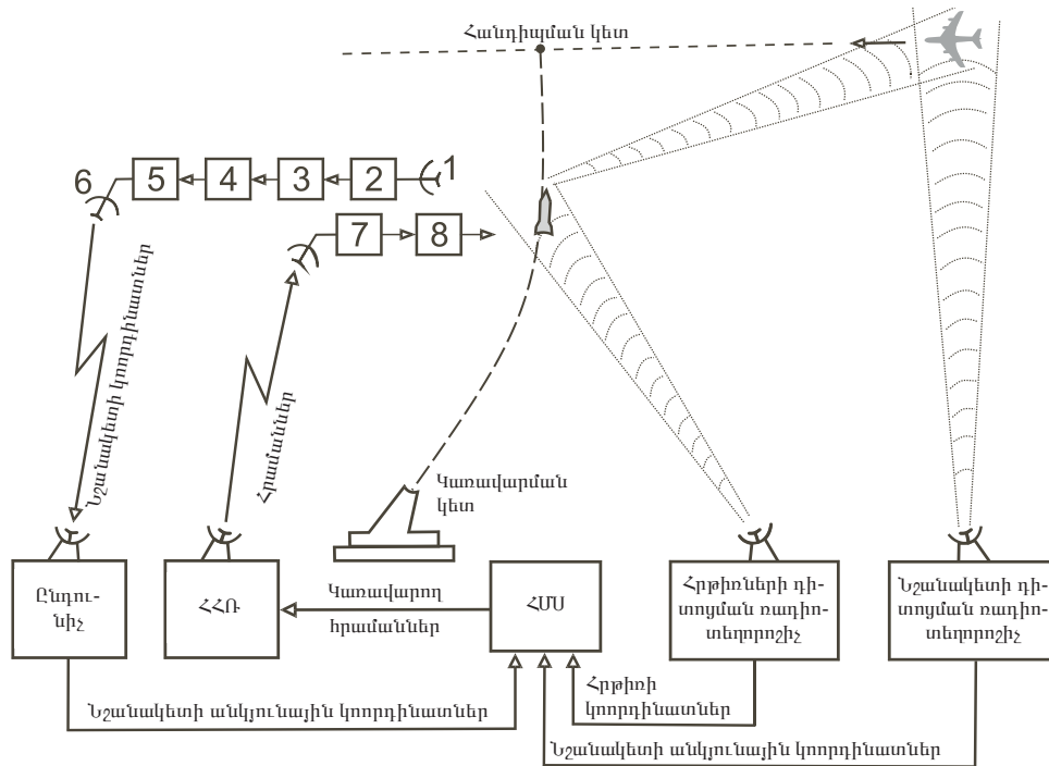
Նկ. 2. Հեռակառավարման համակցված հրամանատու համակարգ
