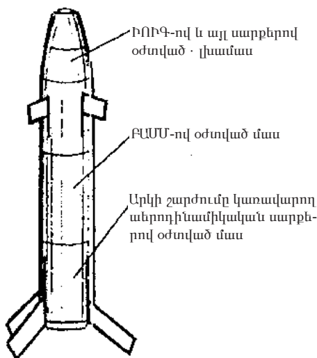
Նկ. 2. 152-մմ կառավարվող 2425 արկ
