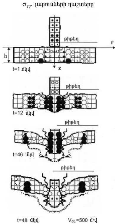
Նկ. 9. V_0 = 720 մ/վ, h = 15 \cdot 10^{-3} մ, J_0 = 10^5 Ա/մ 2
