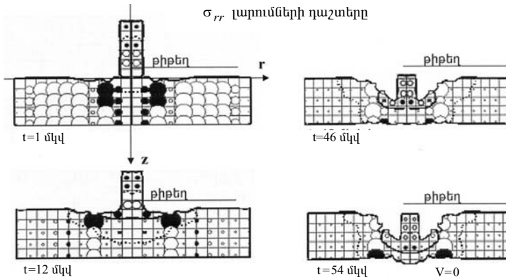
Նկ. 5. V_0=720 \text{ մ}^3/\text{լ} , J_0=10^5 \text{ Ա}/\text{մ}^2
