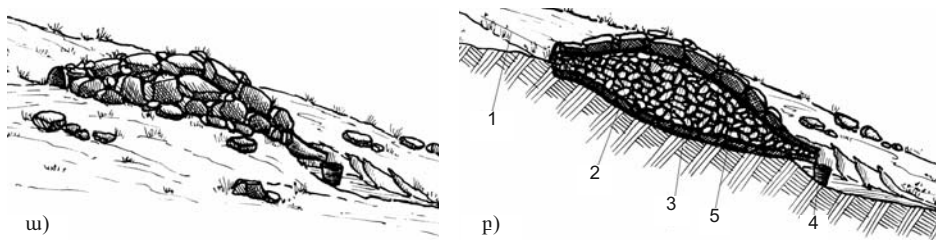
Նկ 2. Խտացման աղբյուրի պարզագույն սխեման ա) ընդհանուր տեսքը, բ) կտրվածքը. 1. մշտապես փչող քամի, 2. խճաքարային լիցք, 3. ջրամբժ շերտ, 4. դույլ՝ խտացված ջուրը հավաքելու համար, 5. բաց գույնի սալիկներ՝ խճաքարի տաքացումը կանխելու համար
