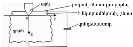
Նկ. 1. Զրահի պաշտպանականության մեծացման էլեկտրադինամիկական մեթոդի գծապատկերը
