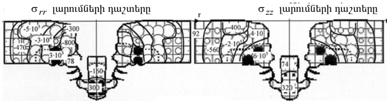
Նկ. 6. Լարումների համապատենցիալ մակերևույթները ( V_0=720 մ/վ, t=62 մկվ, J_0=0 , V_{\text{մն.}}=360 մ/վ (ելքի արագություն))
