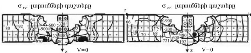
Նկ. 7. V_0=720 մ/վ, t=54 մկվ, J_0=10^5 Ա/մ 2
