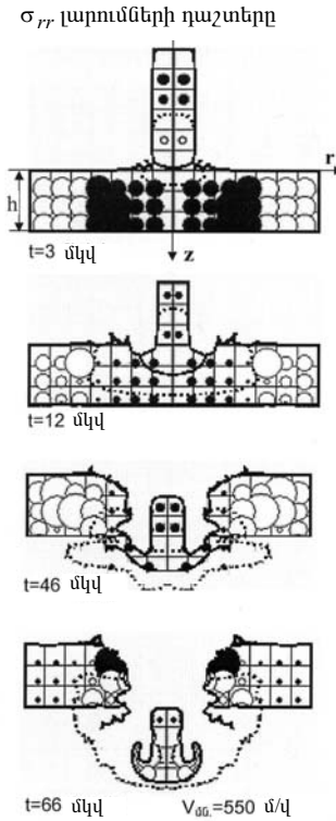
Նկ. 8. V_0 = 720 մ/վ, h = 15 \cdot 10^{-3} մ, J_0 = 0
