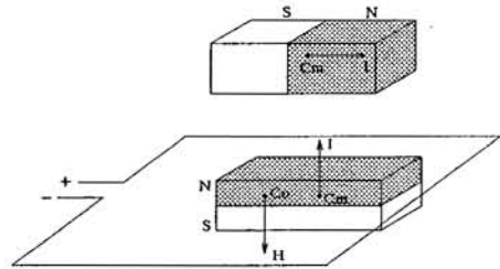
Նկ. 3. Երկայնական մագնիսացման առաջացումը հոսանքով հորիզոնական կոնտուրի ուղղաձիգ մագնիսական դաշտի արդեցությամբ
