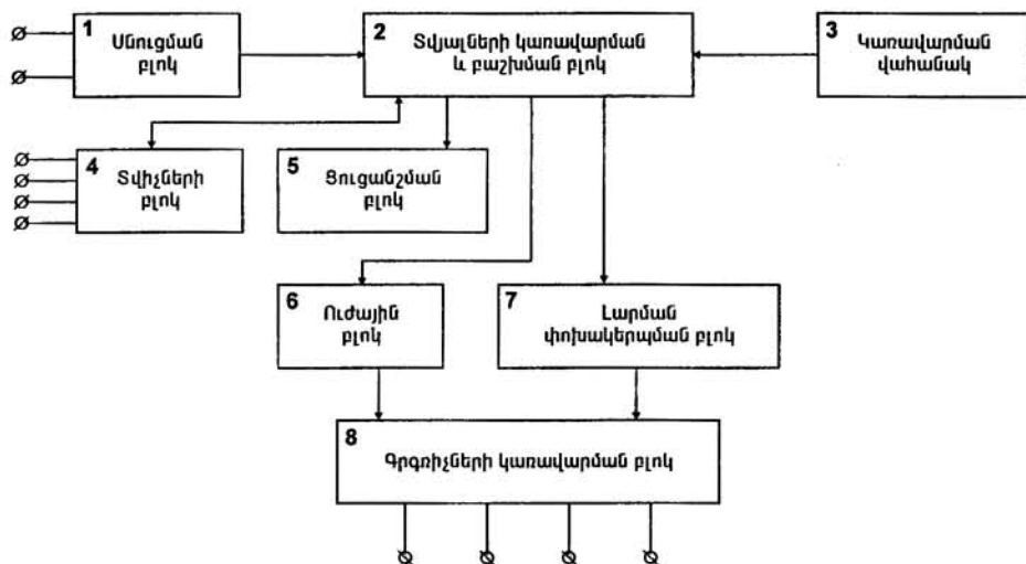
ժամանակային բնութագրերի չափման սարքի բլոկային գծապատկեր
