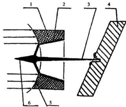
Նկ. 2. Կուտակային շիթի ձևավորման և գրահապատնեջի հետ նրա փոխազդեցության գծապատկեր
