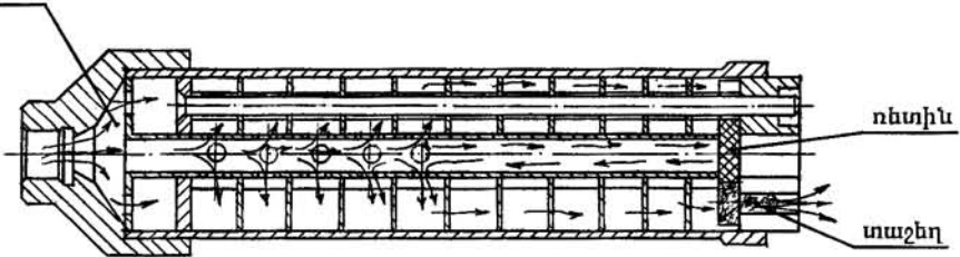
Նկ. 1. Դիֆուզորով խլարարի գծապատկերը
