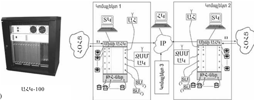
Նկ. 1. Թվային կապի կազմակերպում
