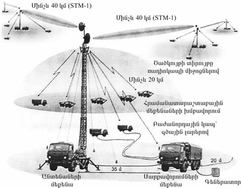
Նկ. 4. Արագ բացազատվող ինտեգրված համակարգ
