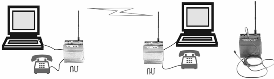
Նկ. 9. Կապի կազմակերպումը ռադիոմոդեմի միջոցով
