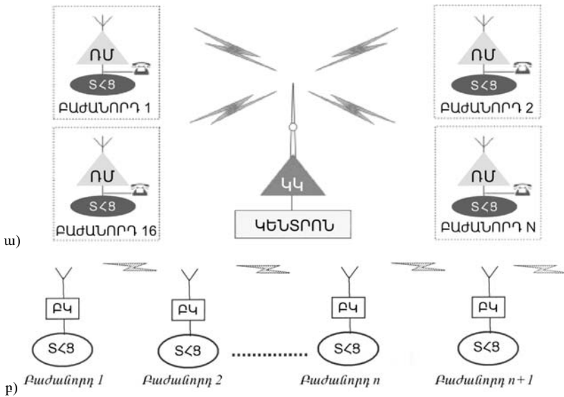
Նկ. 2. Ցանցային ռադիոկապի կազմակերպում
