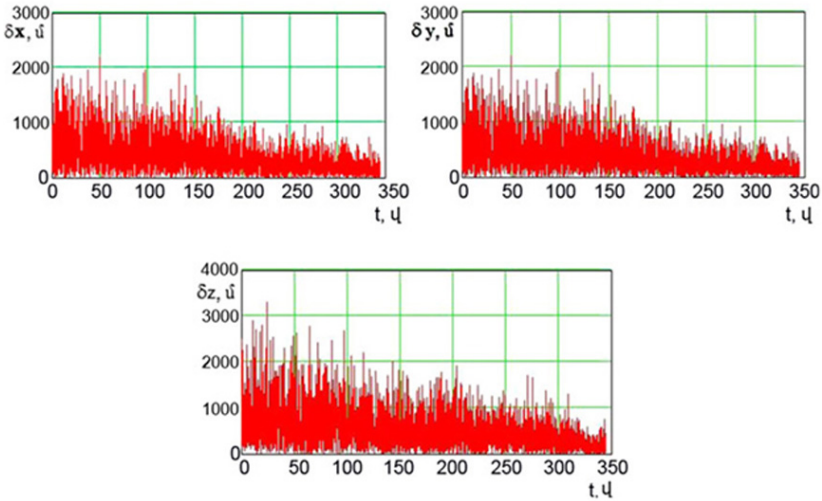
Նկ. 7. Օդային նշանակետի դիտման սխալներն ըստ x , y , z կոորդինատների
