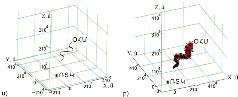
Նկ. 6. ՕՀՄ օձաձև տարաշարժով թռիչքի դիտումը ՈՏԿ-ով.
