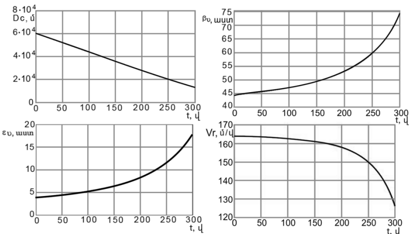
Նկ. 2. Նշանակետի հեռավորությունը, ազիմուտը, տեղի անկյունը, շառավղային արագությունը ՌՏԿ-ի նկատմամբ
