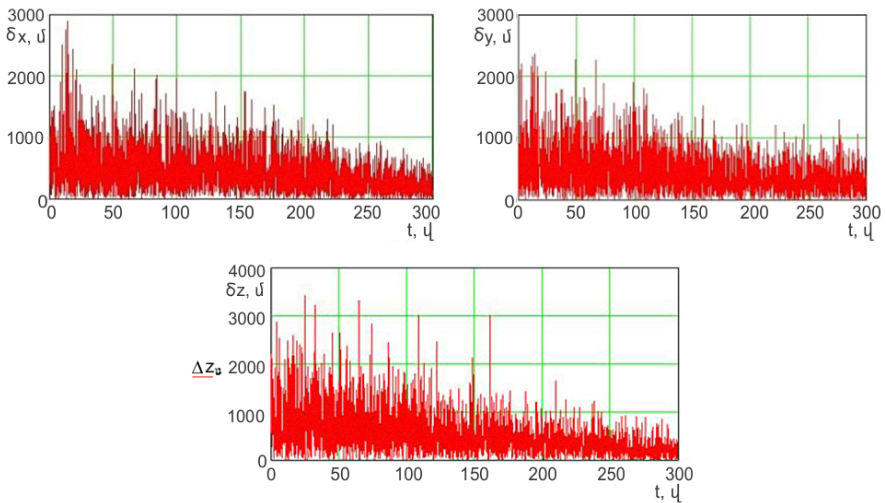
Նկ. 4. Օդային նշանակետի դիտման սխալներն ըստ x, y և z կոորդինատների. օձածն տարաշարժով թռիչքի մոդելավորում
