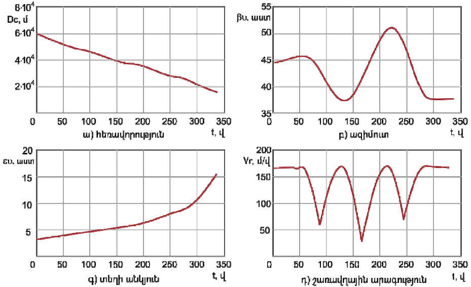
Նկ. 5. Ժամանակի ընթացքում ՕՀՄ պարամետրների փոփոխման գրաֆիկներ
