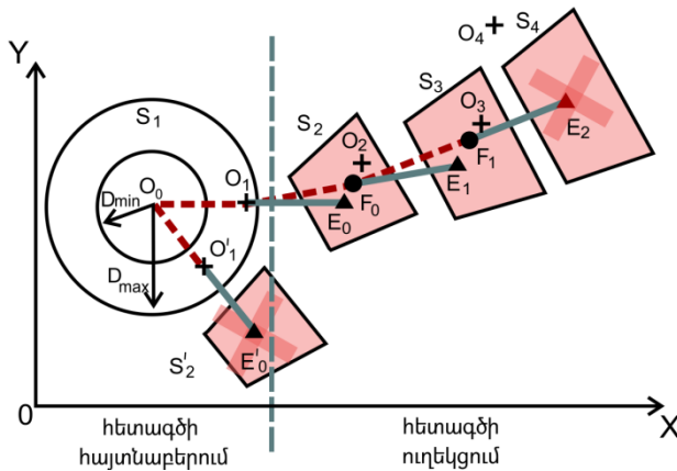
Նկ. 1. Նշանակետի հետագծի հայտնաբերման և ուղեկցման ընթացքը
