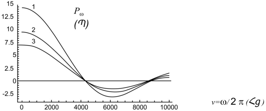
Նկ. 1. ՀՁԱ-ի ճնշման սպեկտրալ կախումը (1՝ h=500 մ, 2՝ h=750 մ, 3՝ h=1000 մ)
