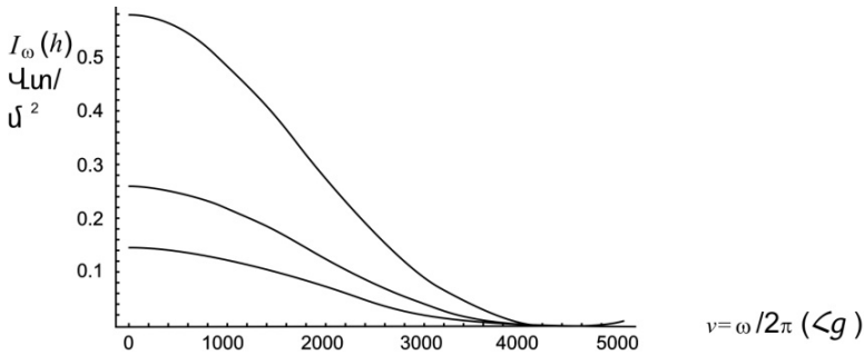
Նկ. 2 ՀՁԱ-ի ինտենսիվության կախումը հաճախականությունից (1՝ h = 500 մ, 2՝ h = 750 մ, 3՝ h = 1000 մ)
