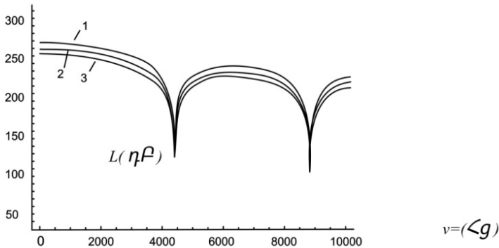
Նկ. 3. Հաճախականությունից ՀՁԱ-ի ինտենսիվության կախումը (1՝ h = 500 մ, 2՝ h = 750 մ, 3՝ h = 1000 մ)
