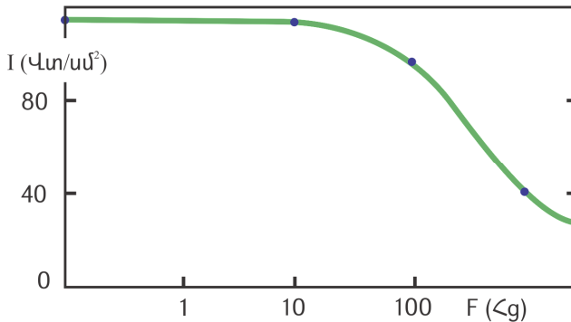
Նկ. 3. Միկրոսխեման վնասելու համար անհրաժեշտ ինտենսիվության կախումը ԳԲՀ իմպուլսների կրկնման հաճախականությունից:
