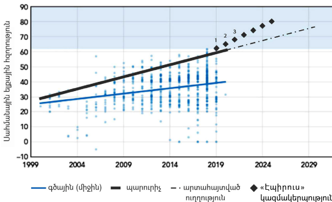
Սկ. 10. Si2-i, GaAs- ի, SiGe- ի, InP- ի և GaN- ի հիման վրա հզորության ուժեղարարների հագեցման հզորությունների աճման 20-ամյա դինամիկան 4 ԳՀց-ից ցածր հաճախական տիրույթում:
