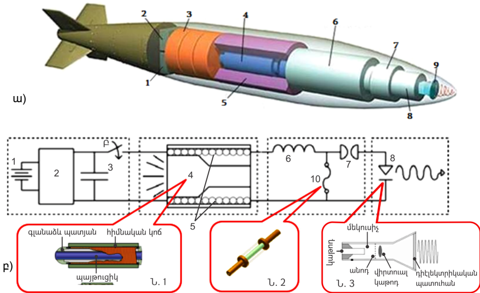
Նկ. 6. Էլեկտրամագնիսական ռուբը. ա) ԷՄՈ-ի կառուցվածքը, բ) ռուբի էլեկտրական սխեման ըստ [3]-ի. 1 – սնուցման աղբյուր, 2 – լարման փոխակերպիչ, 3 – կոնդենսատորային մարտկոց, P – բանալի, 4 – պայթյուցիկ, 5 – հիմնական կոճ, 6 – բալաստային կոճ, 7 – էներգիայի փոխանցման ցանց, 8 – վիրկատոր, 9 – ճառագայթիչ ալեցիր, 10 – ապահովիչ, Ներդիրներ. Ն. 1. – հիմնական զենքատորի կառուցվածքը, Ն. 2. – ապահովիչի կառուցվածքը, Ն. 3. – վիրկատորի կառուցվածքը
