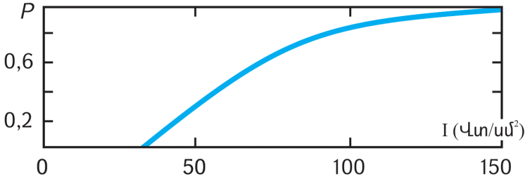
Նկ. 4. Միկրոսխեմայի վնասման հավանականության կախումը 5 մկվ տևողությամբ ռադիոիմպուլսի հզորությունից
