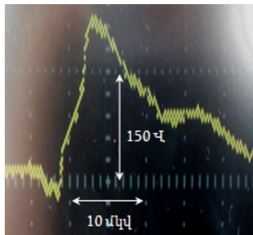
Նկ. 8. 12 մմ տրամագծով մագնիսներով և 6 գալար ունեցող կոճով ԷՄՈ-ով գեներացրած իմպուլսի տատանագիրը
