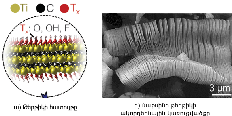
Նկ. 3. Ti_3C_2 մաքսինի թերթիկների պատկերներ
