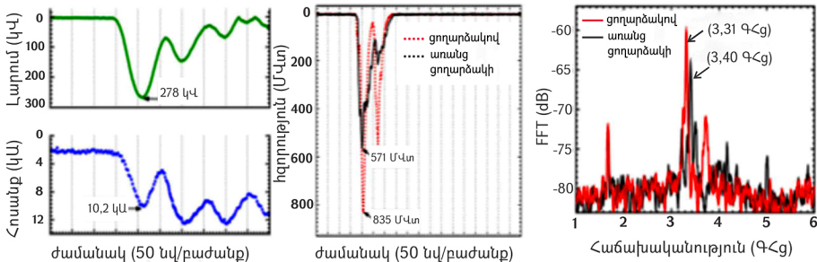
Նկ. 7. Ուղղորդված ճառագայթմամբ վիրկատորի հիմնական պարամետրները
